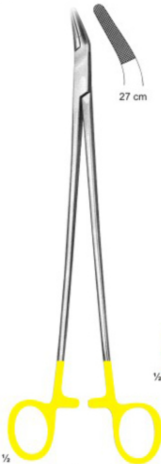
2877 FINOCHIETTO 27 cm
